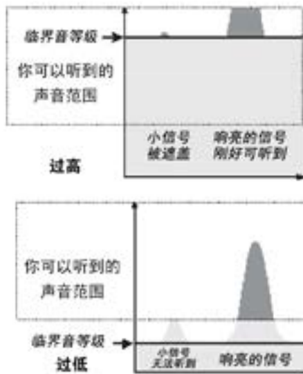
图 17 - 临界音等级
